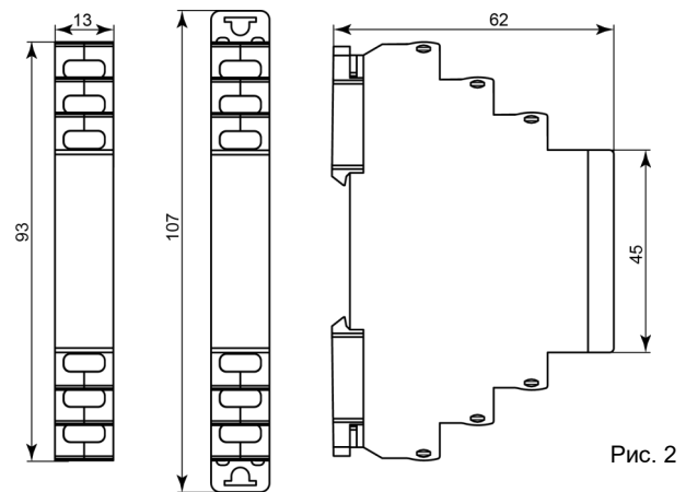
Габаритные размеры
