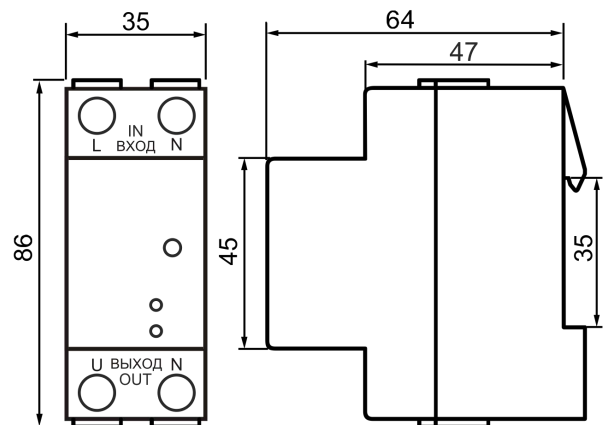
Габаритные размеры
